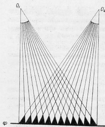
Рис. 6. Параллакс-стереограмма, рассматриваемая на отражение (по П. П. Соколову): O_1 и O_2 — проекционные объективы; \Phi — гофрированный фотослой
