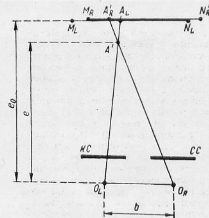
Рис. 2. Схема рассматривания изображения по методу анаглифов: KC — красный светофильтр, через который левый глаз O_L рассматривает синее изображение M_L N_L ; CC — синий светофильтр, через который правый глаз O_R рассматривает красное изображение M_R N_R ; A_R' — точка, рассматриваемая правым глазом на снимке M_R N_R ; A_L — точка, рассматриваемая левым глазом на снимке M_L N_L ; A' — воспринимаемое стереоскопически на расстоянии l от глаза наблюдателя
