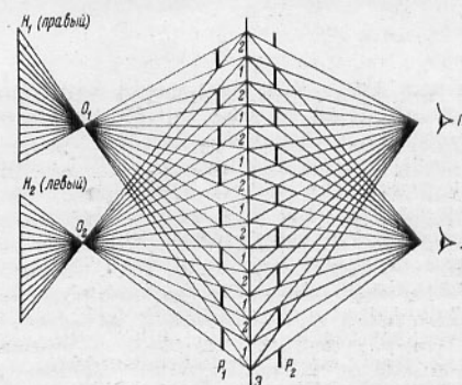
Рис. 5. Замена стереоскопа растром-решеткой: O_1 и O_2 — проекционные объективы; H_1 и H_2 — два кадра стереопозитива; R_1 и R_2 — идентичные растры-решетки; \Theta — экран; L и P — глаза наблюдателя; 1 и 2 — чередующиеся полосы левого и правого изображений
