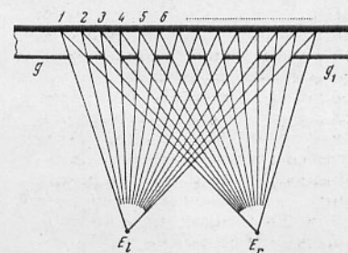
Рис. 3. Схема получения параллакс-стереограммы: E_L и E_R — объективы печатающего устройства; gg_1 — растр-решетка; 1, 2, 3, 4, 5, 6... — изображения стереопары на фотослое, проецируемые объективами E_L и E_R
