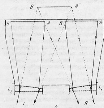
Рис. 1. Линзовый стереоскоп (а) и оптическая схема рассматривания стереопары АВ (б). Наблюдатель воспринимает стереоскопический образ А'В'
